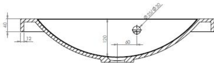
PRZEKRÓJ A-A SKALA 1 : 3
