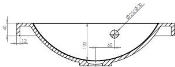
PRZEKRÓJ A-A SKALA 1 : 3
